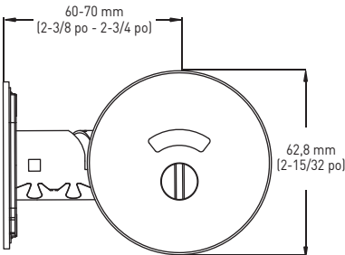
PÊNE DORMANT AVEC INDICATEUR D'OCCUPATION
