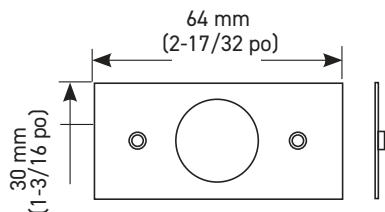
SUPPORT EXTÉRIEUR
