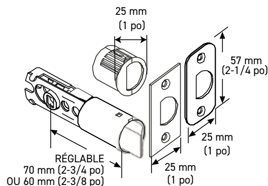
LOQUET 6-EN-1 INTIMITÉ/ PASSAGE
